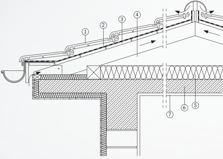
Şekil 1- Çatı arası kullanılmayan eğimli çatılarda ısı yalıtımı
