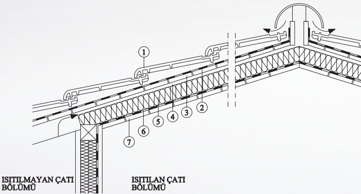
Şekil 2- Çatı arası kullanılan eğimli çatılarda ısı yalıtımı (havalandırılmalı)
